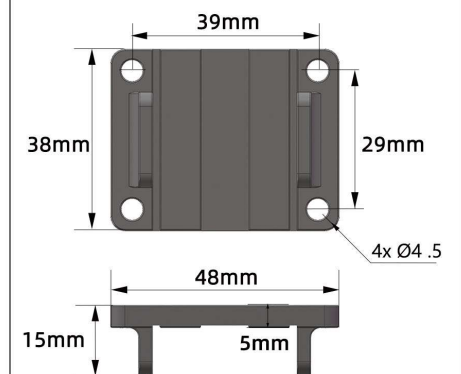
DJ固定地脚尺寸图 / Linear Module Foundation Size
